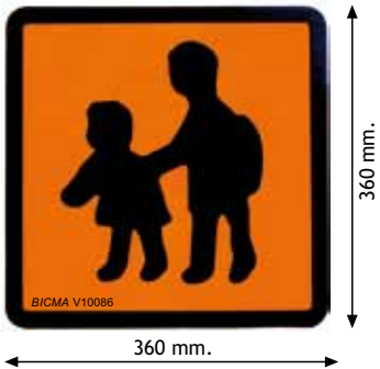
Cod. 80931 Pannello scuolabus alluminio 360x360x1 mm. tipo Spagna pellicola classe 2 Schoolbus panel spanish version aluminium 360x360x1 mm. with film class 2
