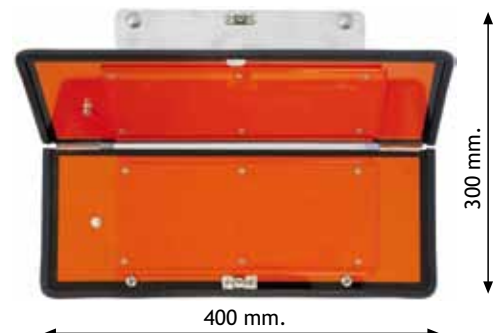
Cod. 92110 Pannello portanumeri inox pieghevole orizzontale 400x300 mm. per numeri 70x118 mm. Horizontal folding stainless steel holder 400x300 mm for numbers 70x118 mm.
