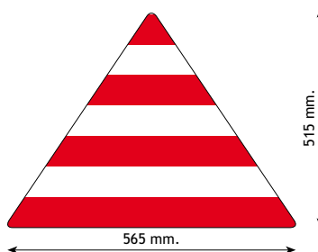
Cod. 70060 Triangolo riflettente per segnalazione posteriore dei trasporti eccezionali Aluminium triangle panel with reflecting film class 1. 565x515x2 mm.
