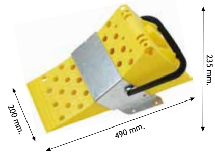
Cod. 95806 Zoccolo fermacamion Omol. DIN 76051 con supporto per zoccolo Wheel chock approved DIN 76051 with holder
