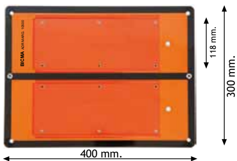
Cod. 91040 Pannello portanumeri inox 400x300 mm. per numeri 70x118 mm. Stainless steel holder 400x300 mm. for numbers 70x118 mm.
